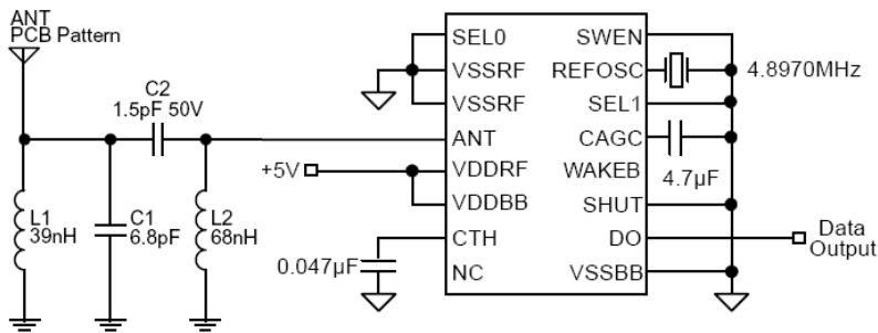
315 MHz 800 bps OOK接收方式
